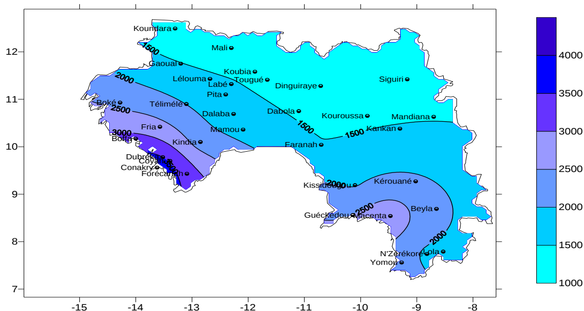
Figure 2 : carte de la pluviométrie moyenne annuelle (1961-2004)
